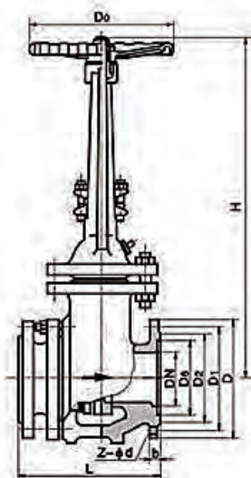
主要外形和连接尺寸(mm)/Main External and Connection Dimension
