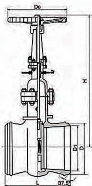
主要外形和连接尺寸Main External and Connection Dimension
